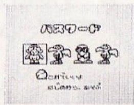
がめん (画面3)
